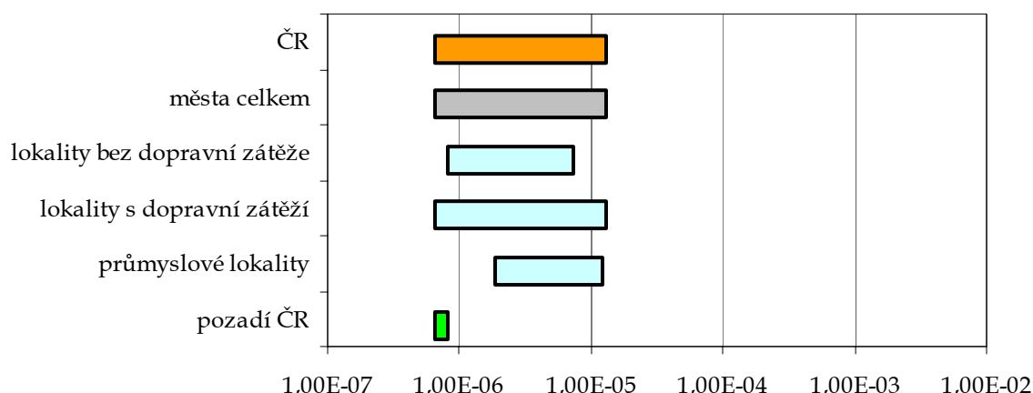
Srovnání rozpětí teoretického odhadu pravděpodobnosti zvýšení počtu nádorových onemocnění z příjmu As z venkovního ovzduší v roce 2008 v ČR a pro jednotlivé typy městských lokalit
