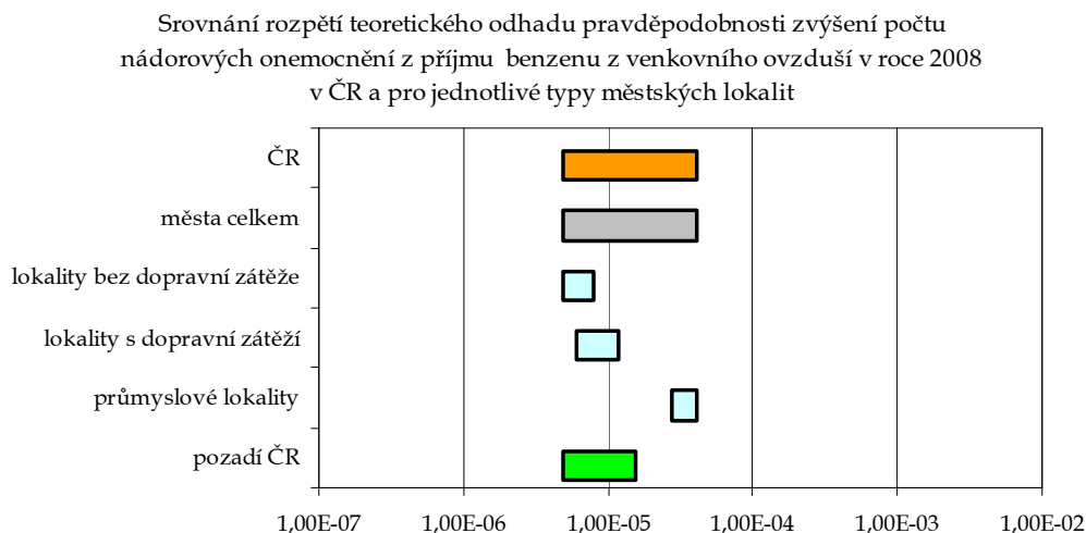
Graf č. 6. - Srovnání rozpětí teoretického odhadu pravděpodobnosti zvýšení počtu nádorových onemocnění z příjmu benzenu z venkovního ovzduší v roce 2008 v ČR a pro jednotlivé typy městských lokalit
