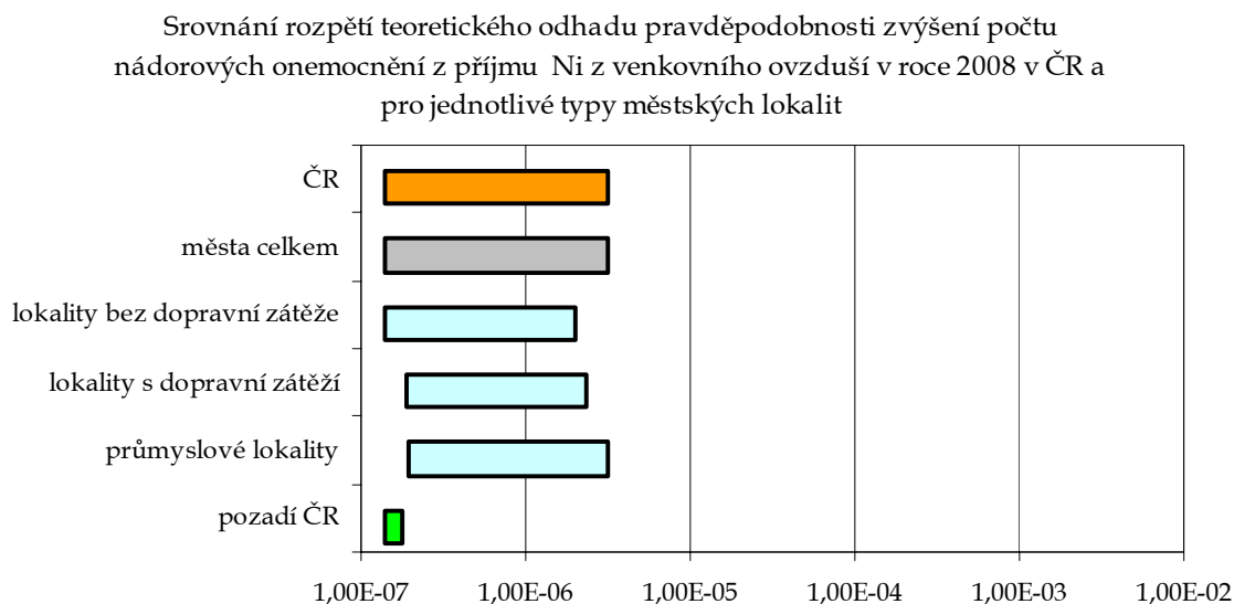
Graf č. 5. - Srovnání rozpětí teoretického odhadu pravděpodobnosti zvýšení počtu nádorových onemocnění z příjmu Ni z venkovního ovzduší v roce 2008 v ČR a pro jednotlivé typy městských lokalit
