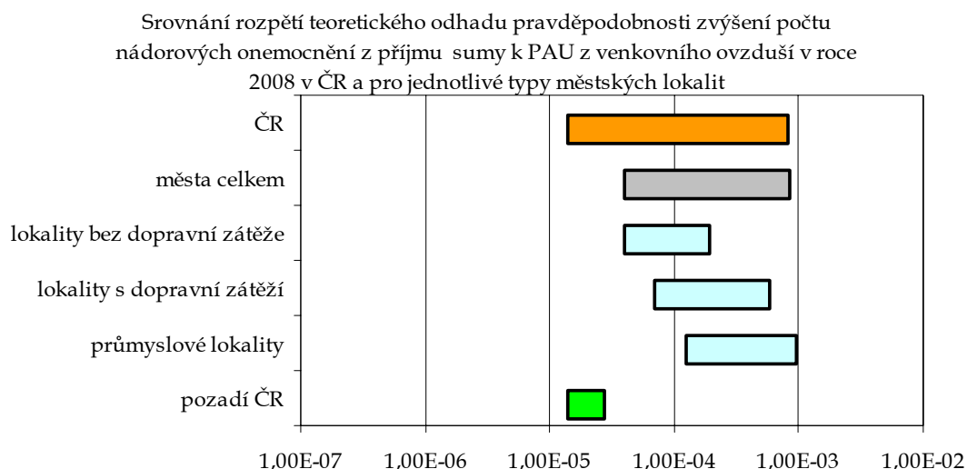
Graf č. 7. - Srovnání rozpětí teoretického odhadu pravděpodobnosti zvýšení počtu nádorových onemocnění z příjmu sumy k PAU z venkovního ovzduší v roce 2008 v ČR a pro jednotlivé typy městských lokalit
