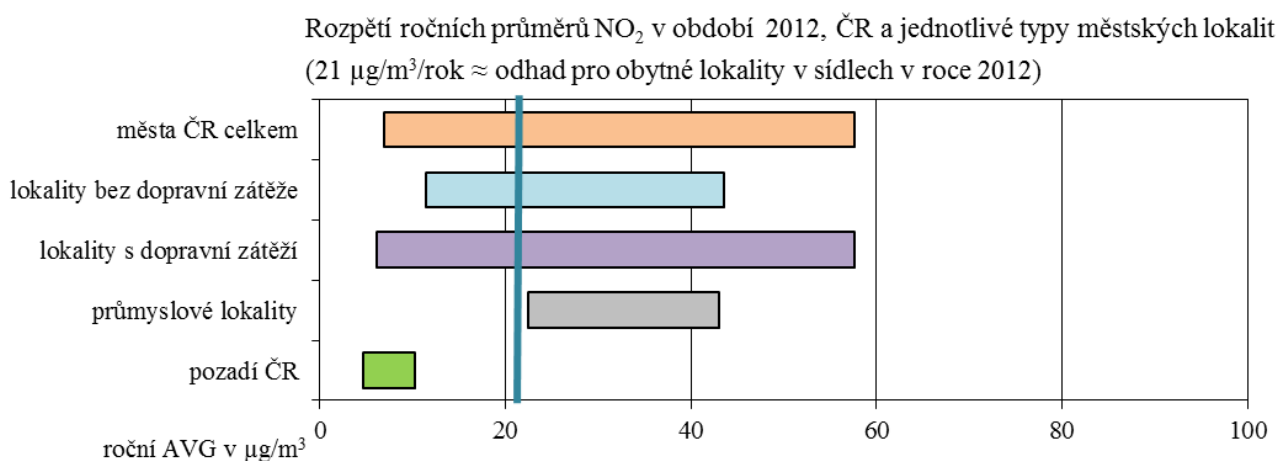
Graf č. 1. Rozpětí ročních průměrů NO 2 v roce 2012 v ČR a v jednotlivých typech městských lokalit
