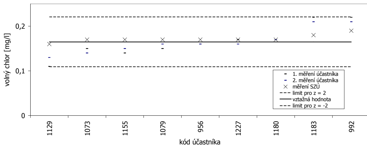
Obrázek 2: Měření volného chloru – umělý vzorek
